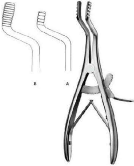
MI-7507 Mouth Gag
